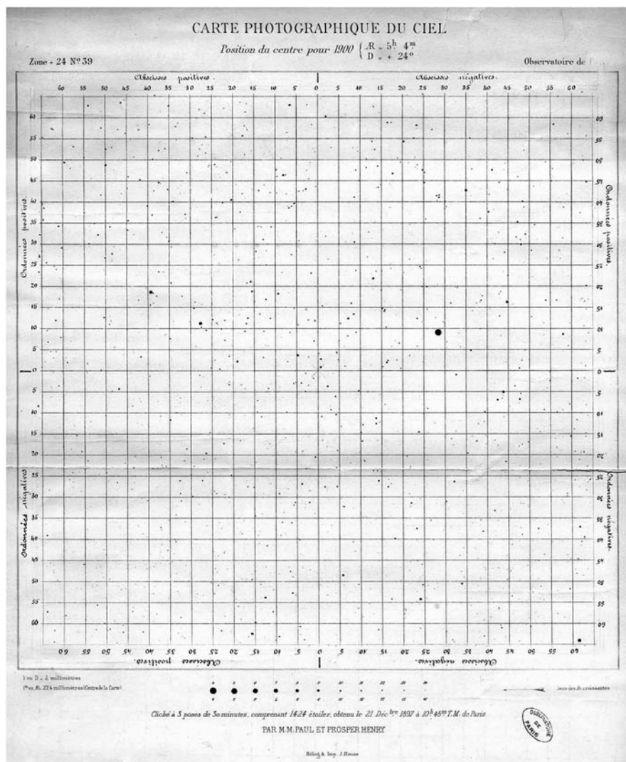
Fig. 6.3 Héliogravure proof of a Carte du Ciel photographic plate. Bibliothèque de l'Observatoire de Paris.
